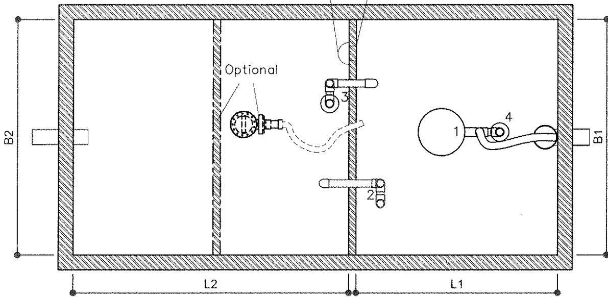
Schlamm Speicher/ Puffer (SP) Belebungsraum (SBR) Tauchwand (optional) Notüberlauf
